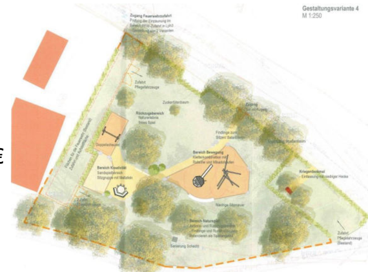
Freianlagenplan Grundschule Klaffenbach
