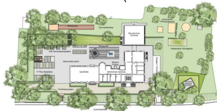
Freianlagenplan Grund- und Oberschule Schönau
